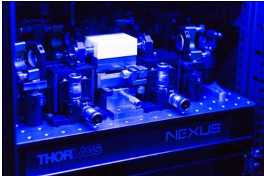
Realer Aufbau
